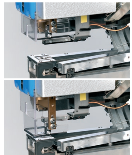
Bewegliches (aktives) Fingerschutzsystem Große Durchlasshöhe und Einlegetiefe im Ansetzbereich
