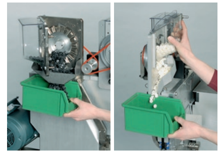
2 Artikelmagazine mit Entleerungssystem Two hopper systems with emptying system
