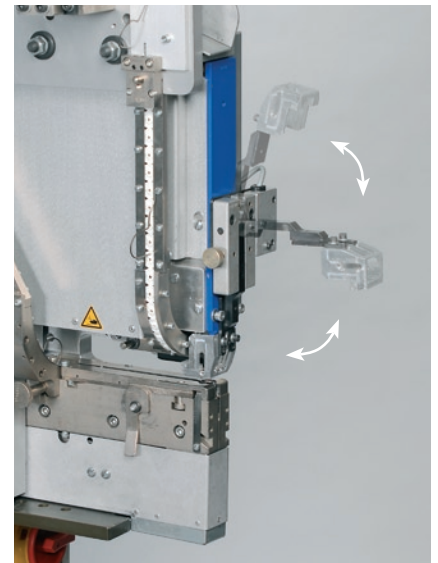
Starres (passives) Fingerschutzsystem Große Einlegetiefe im Ansetzbereich Fixed (passive) finger guard system Great throat depth in the setting area
