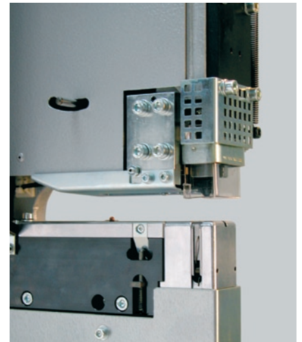
Bewegliches (aktives) Fingerschutzsystem Große Durchlasshöhe und Einlegetiefe im Ansetzbereich
