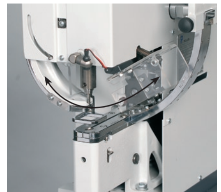
Große Ausladung (Einlegetiefe), frei drehbarer Fingerschutzbügel Great throat depth, rotatable finger guard
